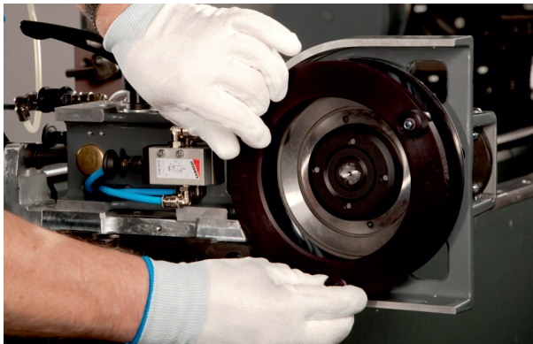
Remplacement du couteau supérieur à changement rapide équipé du protège-lame Valmet. Les 4 vis en acier visibles attestent que la bague de retenue est en place et verrouillée.
