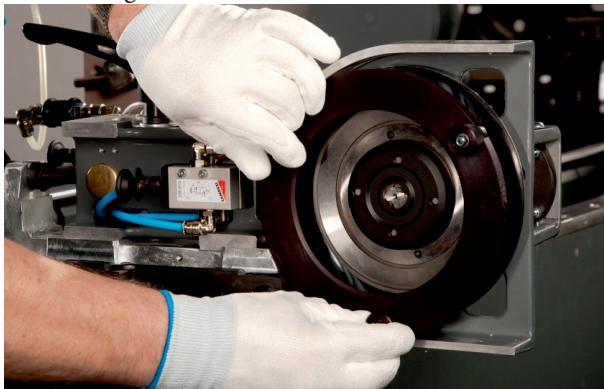
Der Schnellwechsel des Obermessers nutzt einen Schutzring. Die vier erkennbaren Stahlstifte zeigen an, dass der Verriegelungsring in Position und arretiert ist.
